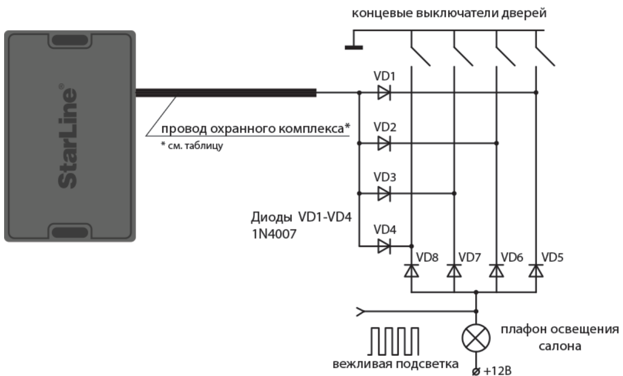
Схема светодиаодной развязки для концевых выключателей отрицательной полярности
